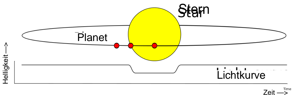
Abbildung 1: Wenn ein Planet vor seinem Stern vorbeiwandert, wird auf der Erde weniger Licht empfangen. Dies ist die Transit-Methode zur Entdeckung von Exoplaneten.
