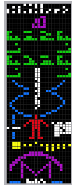
Abbildung 4: Arecibo-Botschaft
