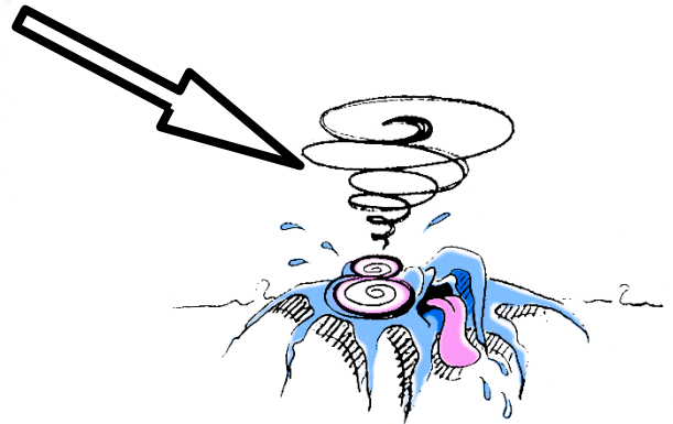
Ein schnell rotierender Neutronenstern - Meike Weisner
