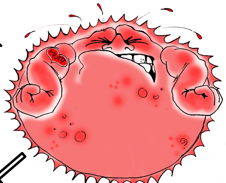
Roter Riese - Meike Weisner
