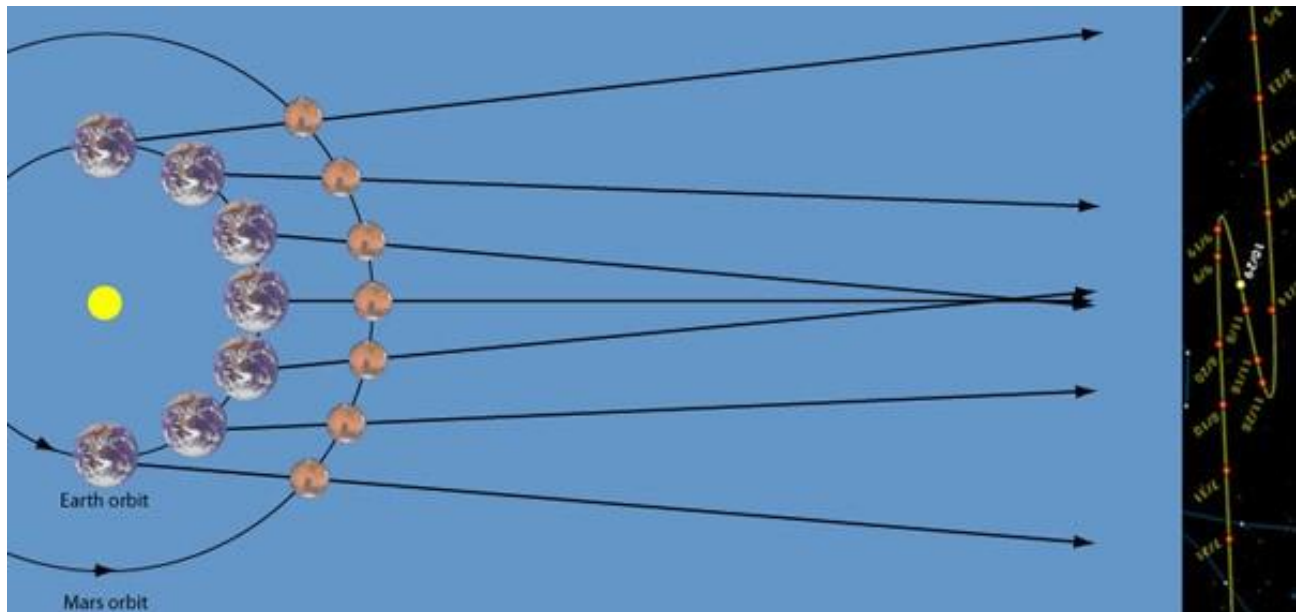
Abbildung 8: Wenn die Erde auf der Innenbahn den Mars überholt, sieht es von der Erde
